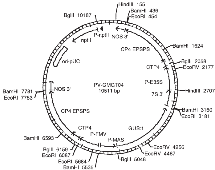
Figura 1. Mapa del plásmido PV-GMGT04 utilizado para producir la soja Roundup Ready, evento 40-3-2.
