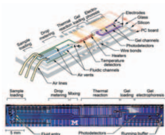
Fig. 8. Dispositivos microelectrónicos Lab-on-a-chip. M.Krishnan, V. Namasivayam, R. Lin, R.Pal, M.A. Burns. Curr. Op. Biotech. 2001, 12, 92-98.
